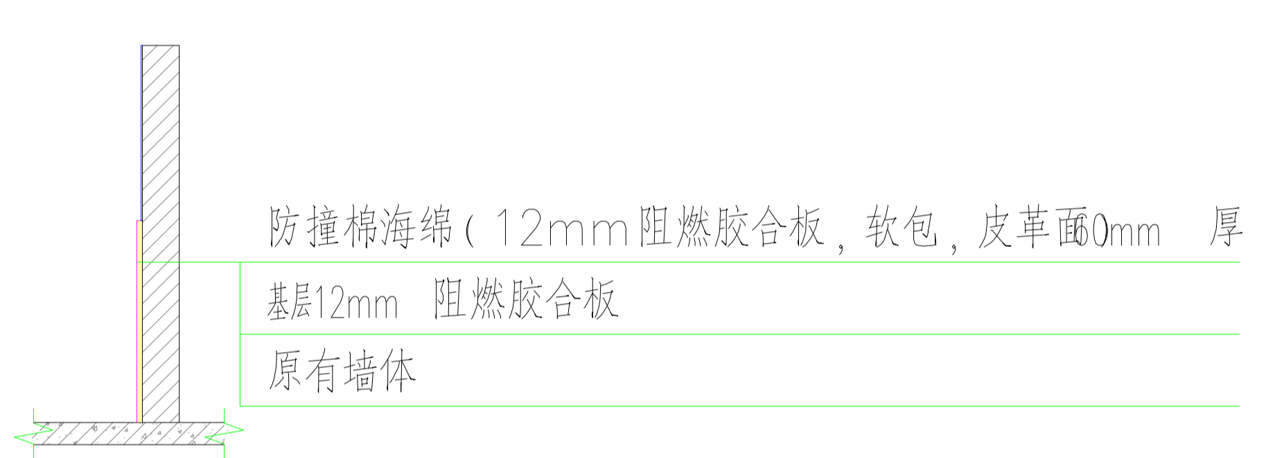
墙裙安装大样图
